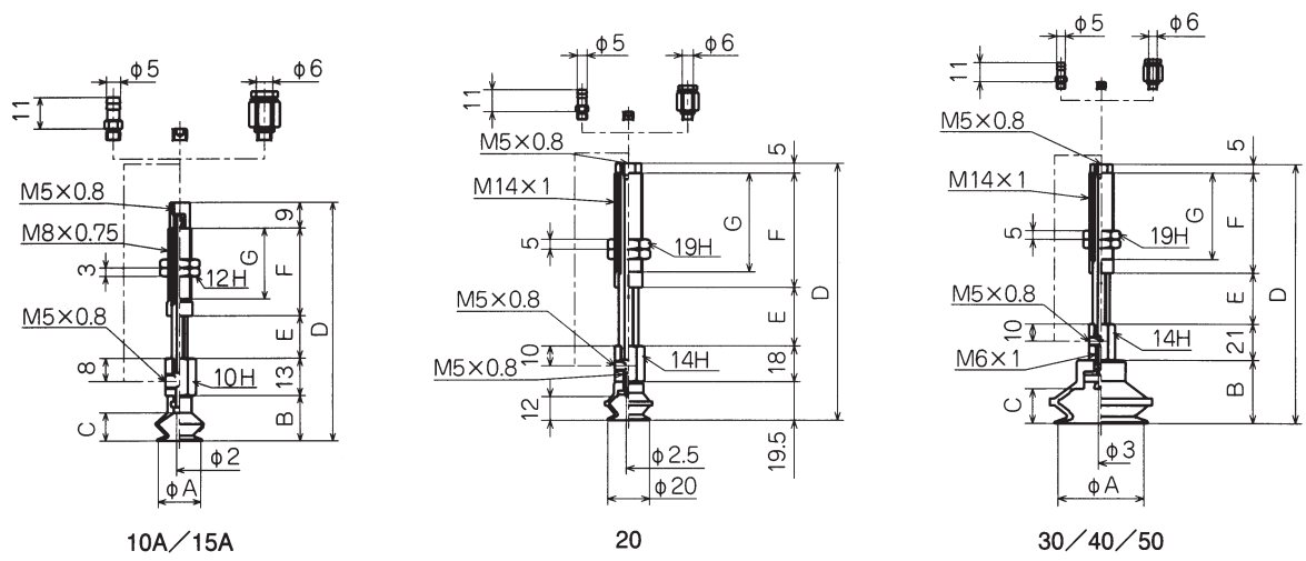
外形尺寸图
