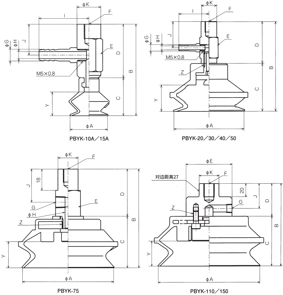
外形尺寸图
