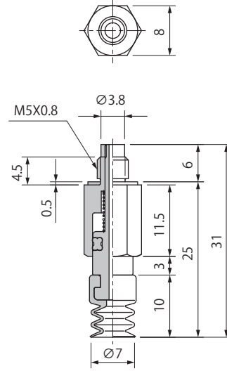
PSS-L3-PCG-7
