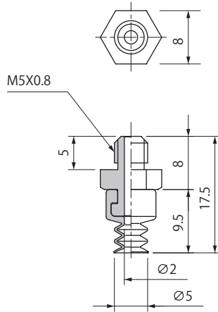
PS-5-C-M
