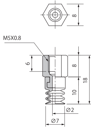
PS-7-C-F
