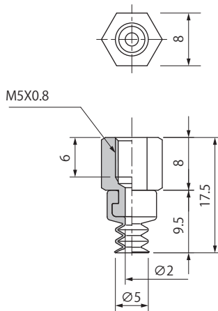
PS-5-C-F
