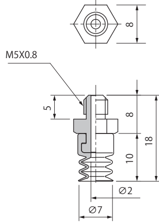
PS-7-C-M
