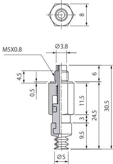
PSS-L3-PCG-5
