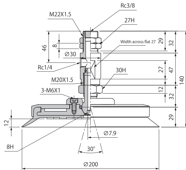
Side Port PUYKB-200
