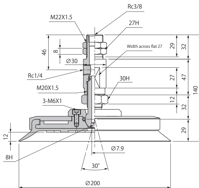
Top Port PUTKB-200
