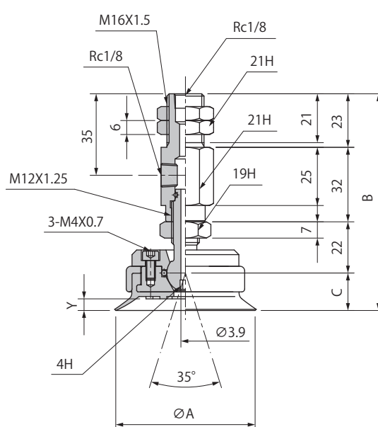
Top Port PUTKB-60 / 80 / 100
